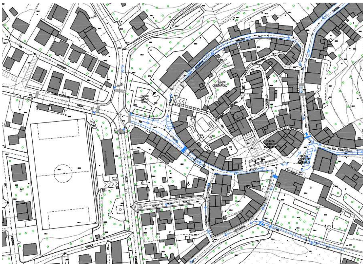
Estratto elaborato grafico PIANO URBANO DEL TRAFFICO Bettolle centro – STATO DI PROGETTO: a cura di R.T.P. – Corsi, Marzi, Monachini
